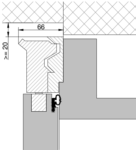
6.1. Ohne Abdeckwinkel / sans équerre
