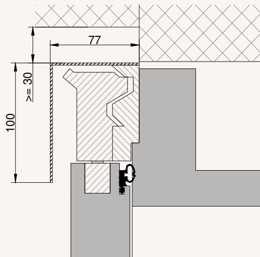
6.2. mit Abdeckwinkel / avec équerre
