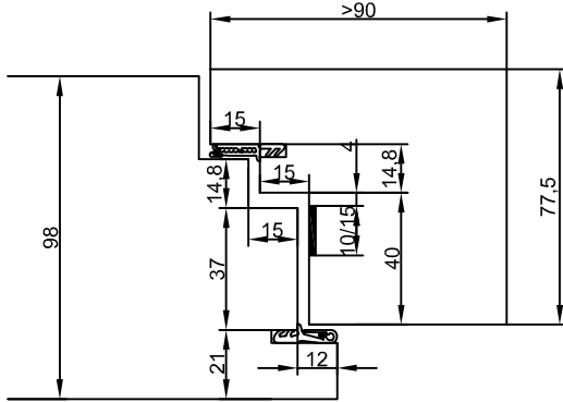
ClimaTop Plus MBW / LBW / PM / PL COMBIModul Blendrahmen / Cadre applique
