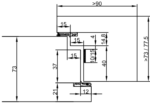
ClimaTop Eco MBW / LBW / PM / PL COMBIModul Blendrahmen / Cadre applique
