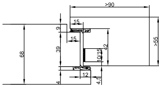
MBW / LBW / PM / PL CombiModul Blendrahmen Cadre applique
