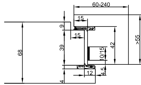
MBW / LBW / PM / PL CombiModul Blockrahmen Cadre bloc
