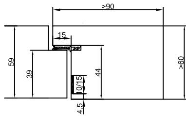
CombiModul Blendrahmen / Cadre applique
