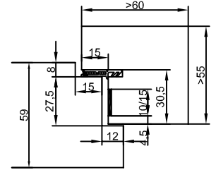
CombiModul Blockrahmen / Cadre bloc reduzierte Falztiefe; 1-flg; ohne Glas, / Profondeur battue réd.; 1 vantaill; sans verre max. 1050 x 2200mm
