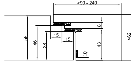
CombiModul Blendrahmen Doppelfalz, nicht für alle Schwellen verfügbar Cadre applique double battue; non applicable pour tous les types de seuils
