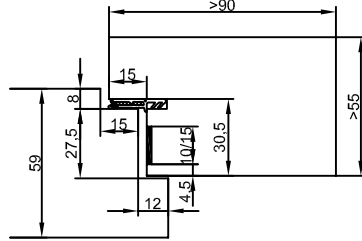
CombiModul Blendrahmen / Cadre applique reduzierte Falztiefe; 1-flg; ohne Glas, / Profondeur battue réd.; 1 vantaill; sans verre max. 1050 x 2200mm
