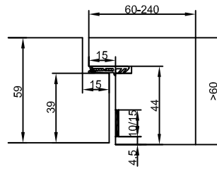
CombiModul Blockrahmen / Cadre bloc
