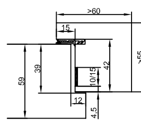
CombiModul Blockrahmen / Cadre bloc
