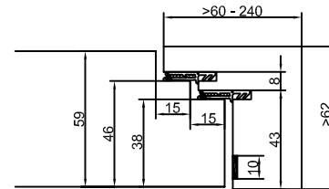
CombiModul Blockrahmen Doppelfalz, nicht für alle Schwellen verfügbar Cadre applique double battue; non applicable pour tous les types de seuils
