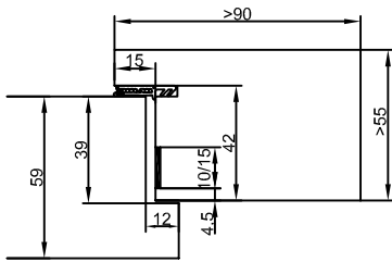
CombiModul Blendrahmen / Cadre applique
