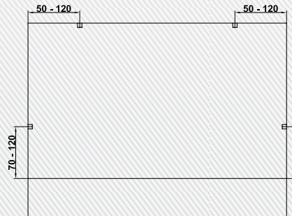
Oberblende Positionierung Aluwinkel
