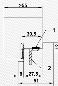
CombiModul überfälzt Vertikal- und Horizontalschnitt Oberblende - Rahmen
