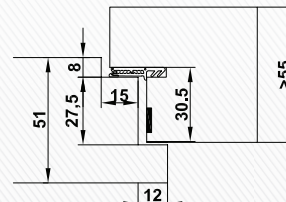
CombiModul überfälzt Horizontalschnitt Türblatt - Rahmen
