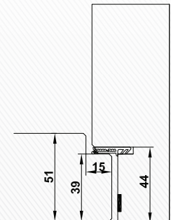
BLOCTool Horizontalschnitt Türblatt - Rahmen
