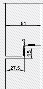
Vertikalschnitt Türblatt / Oberblende überfälzt
