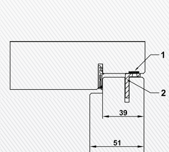
BLOCTool Vertikal- und Horizontalschnitt Oberblende - Rahmen
